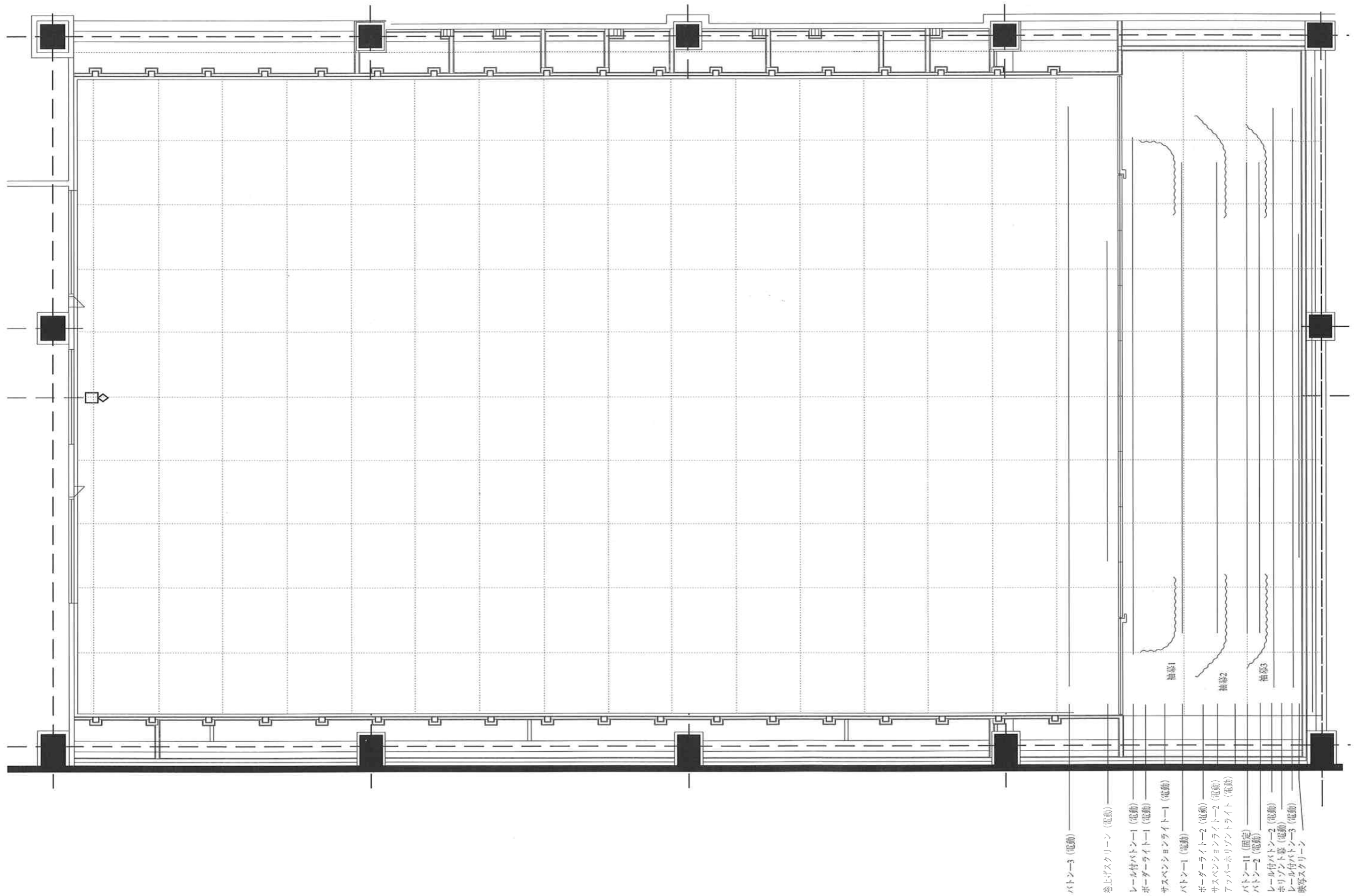
エルガーラホール (8F大ホール) 平面配置図 舞台 1/100
